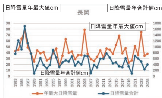
図5 日降雪量の年合計値と日降雪量の年最大値の経年変化(長岡)
