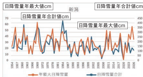
図4 日降雪量の年合計値と日降雪量の年最大値の経年変化(新潟)
